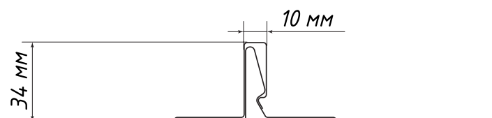
Замок
